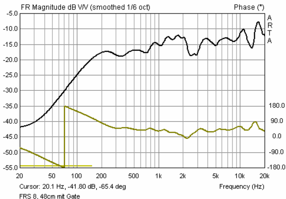
Bild 11: gefensterter Quasi-Freifeldfrequenzgang
