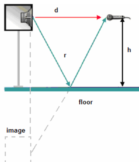
Bild 15: Messaufbau zur Ermittlung des Frequenzgangs
