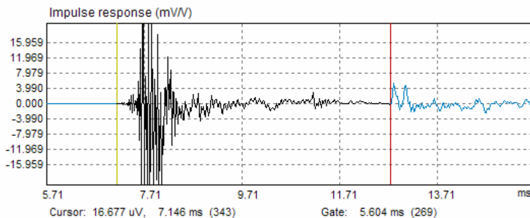
Bild 10: Impulsantwort in 48 cm mit Gate von 5,604 ms
