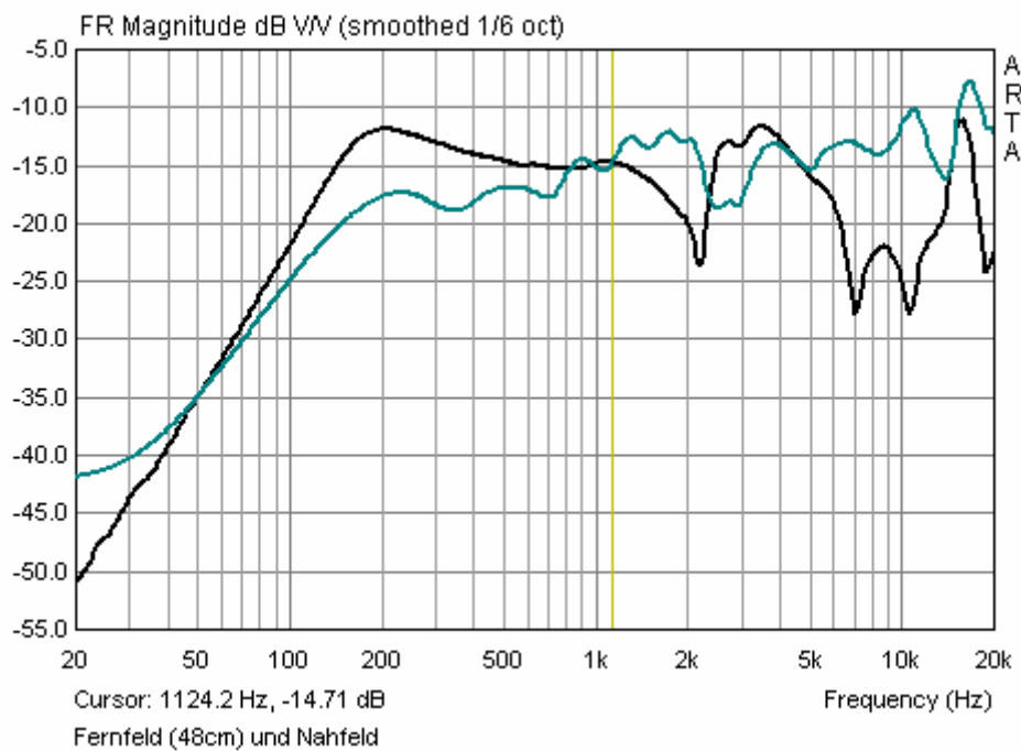
Bild 12: gefensterter Quasi-Freifeldfrequenzgang (grünblau) und Nahfeldfrequenzgang (schwarz)
