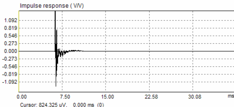
Bild 1: Impulsantwort eines Lautsprechers im normalen Wohnraum. Mikrofon direkt vor der Lautsprechermembran (Nahfeld)
