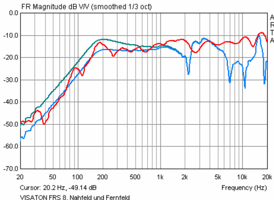
Bild 9: Nahfeldfrequenzgang auf 48 cm skaliert (blaugrün), mit Baffle Step Equalizer korrigiert (hellblau) und Fernfeldfrequenzgang (rot) in 48 cm
